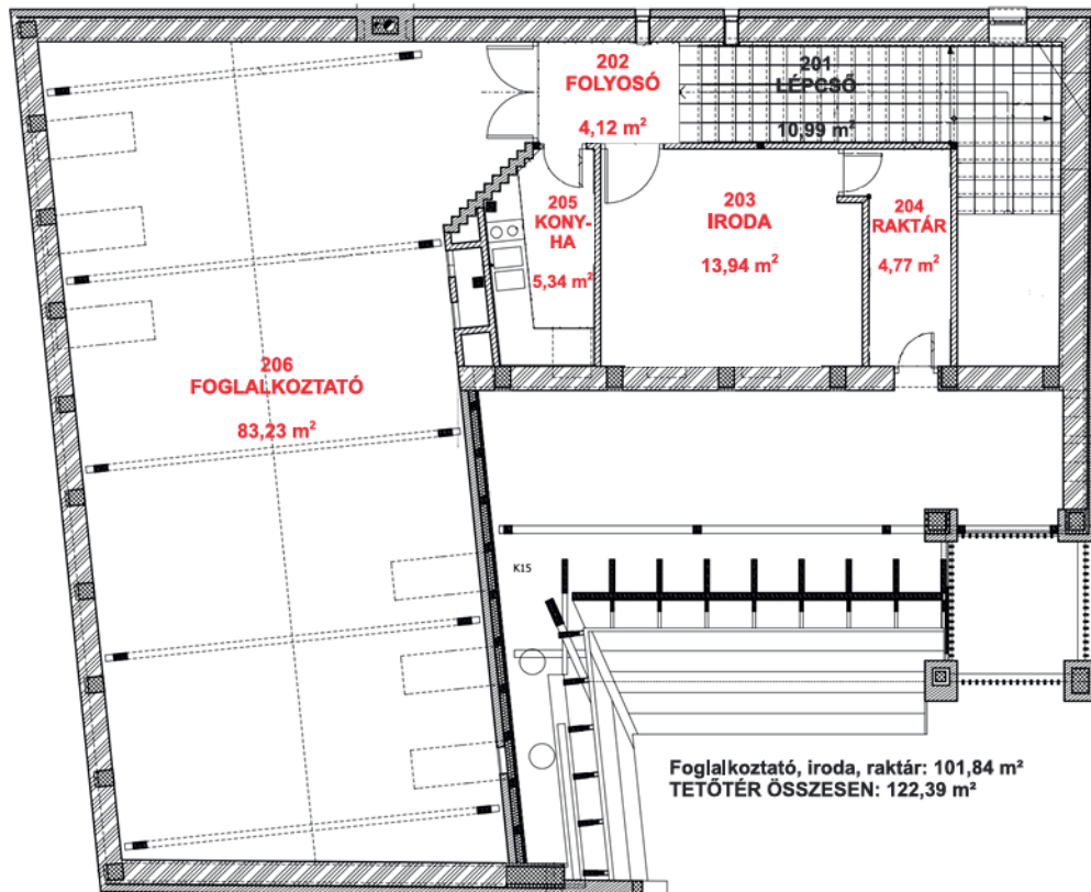
RÁKÓCZI FERENC UTCA 14. TETŐTÉR ALAPRAJZ
